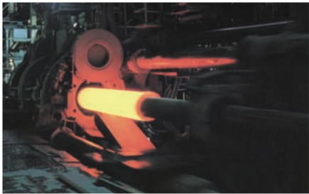
熱間押抜製管機 Horizontal push bench
