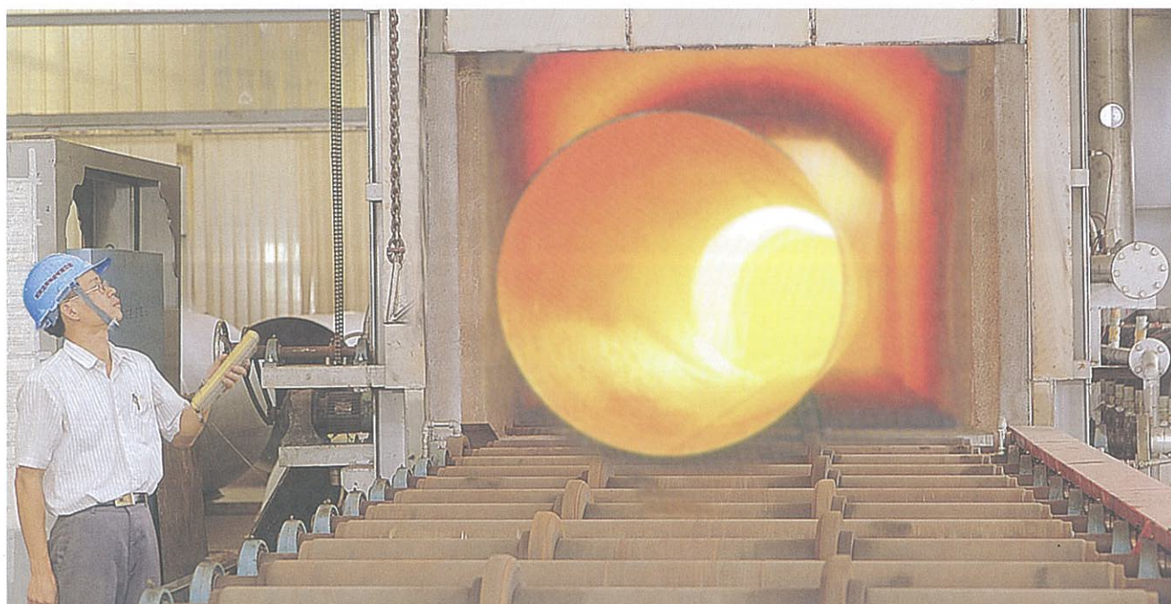
固溶化熱處理設備 solution annealing furnace
