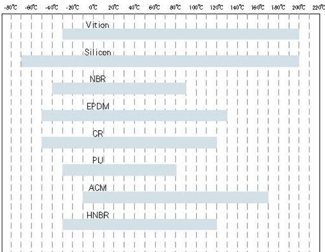
橡膠耐高低溫範圍
