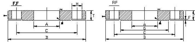
ANSI 150型 FLANGES
