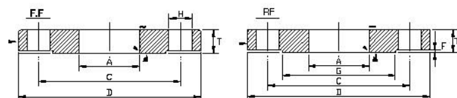
ANSI 300型 FLANGES
