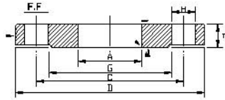
ANSI 125型 FLANGES
