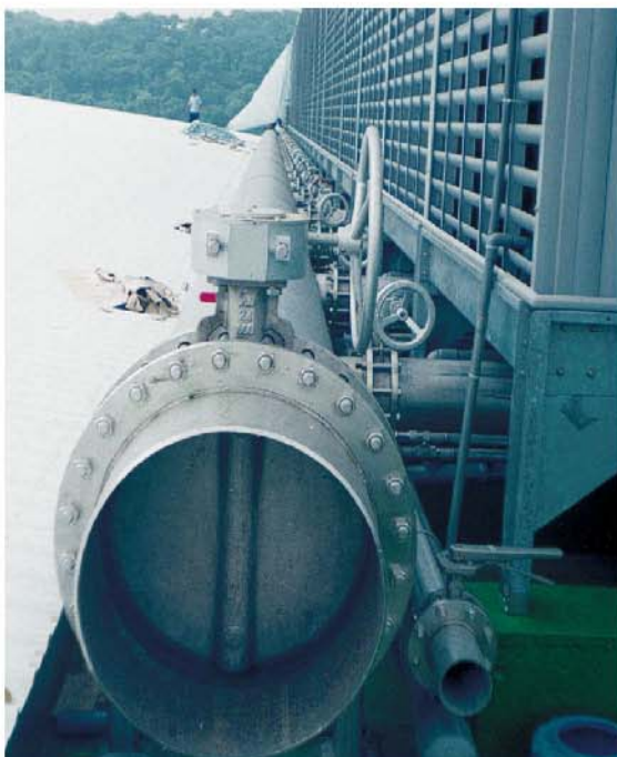
24"不銹鋼蝶閥使用實例
