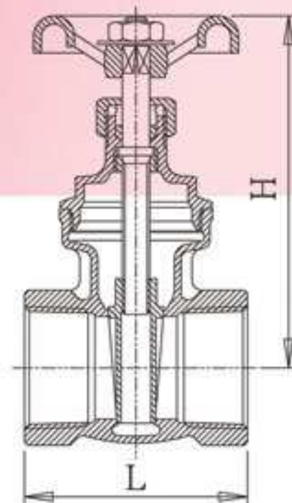
FIG.B01(螺紋口) FIG.B05(法蘭口)
