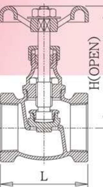
FIG.B11(螺紋口) FIG.B13(法蘭口)
